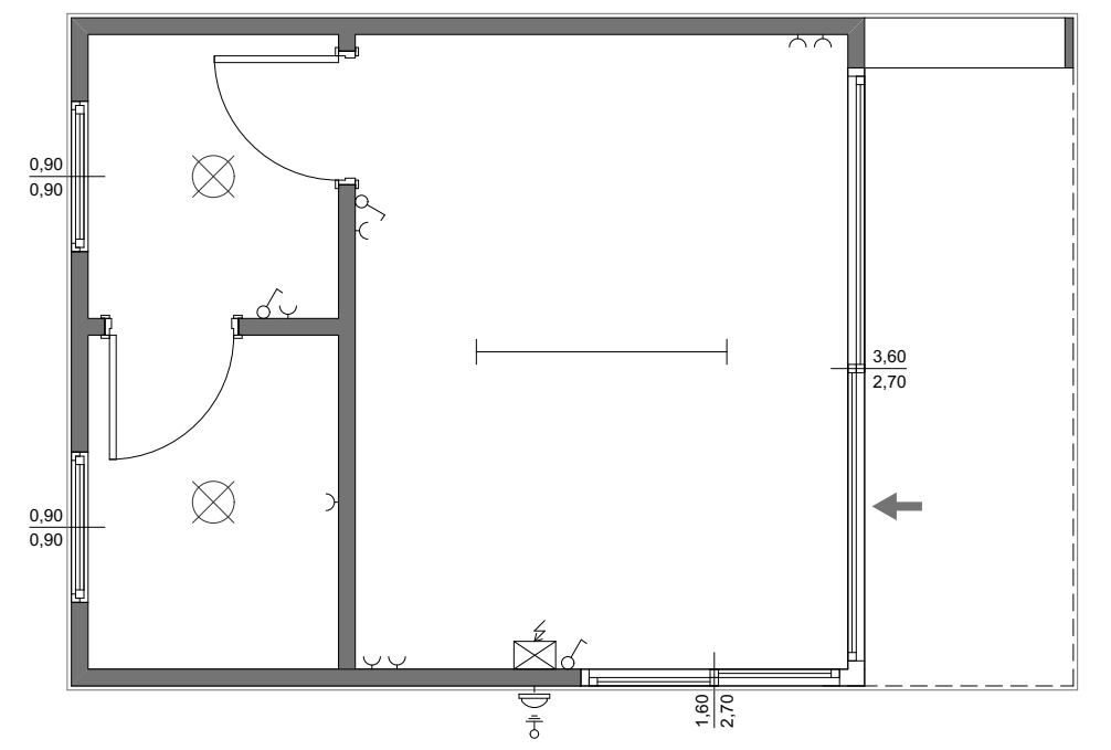
Pianta ufficio - schema elettrico
