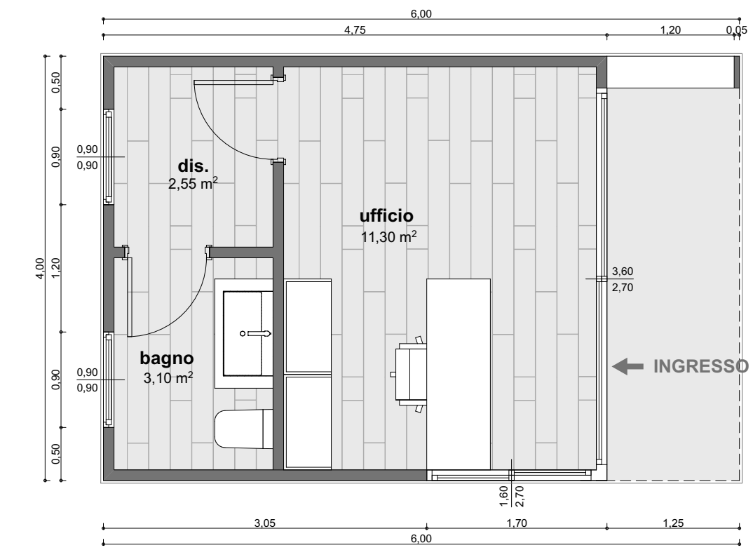
Pianta ufficio
