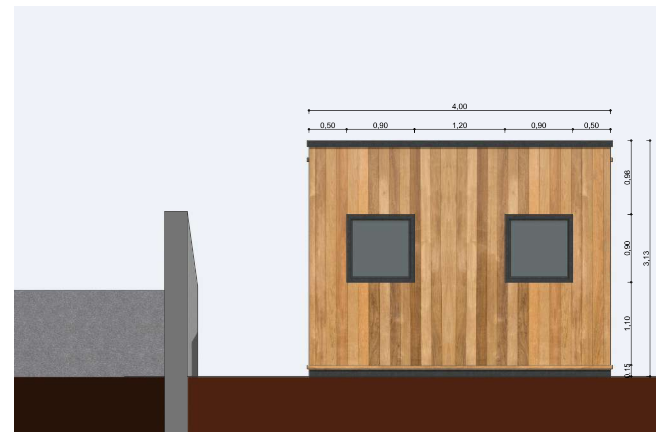
Prospetto SUD
