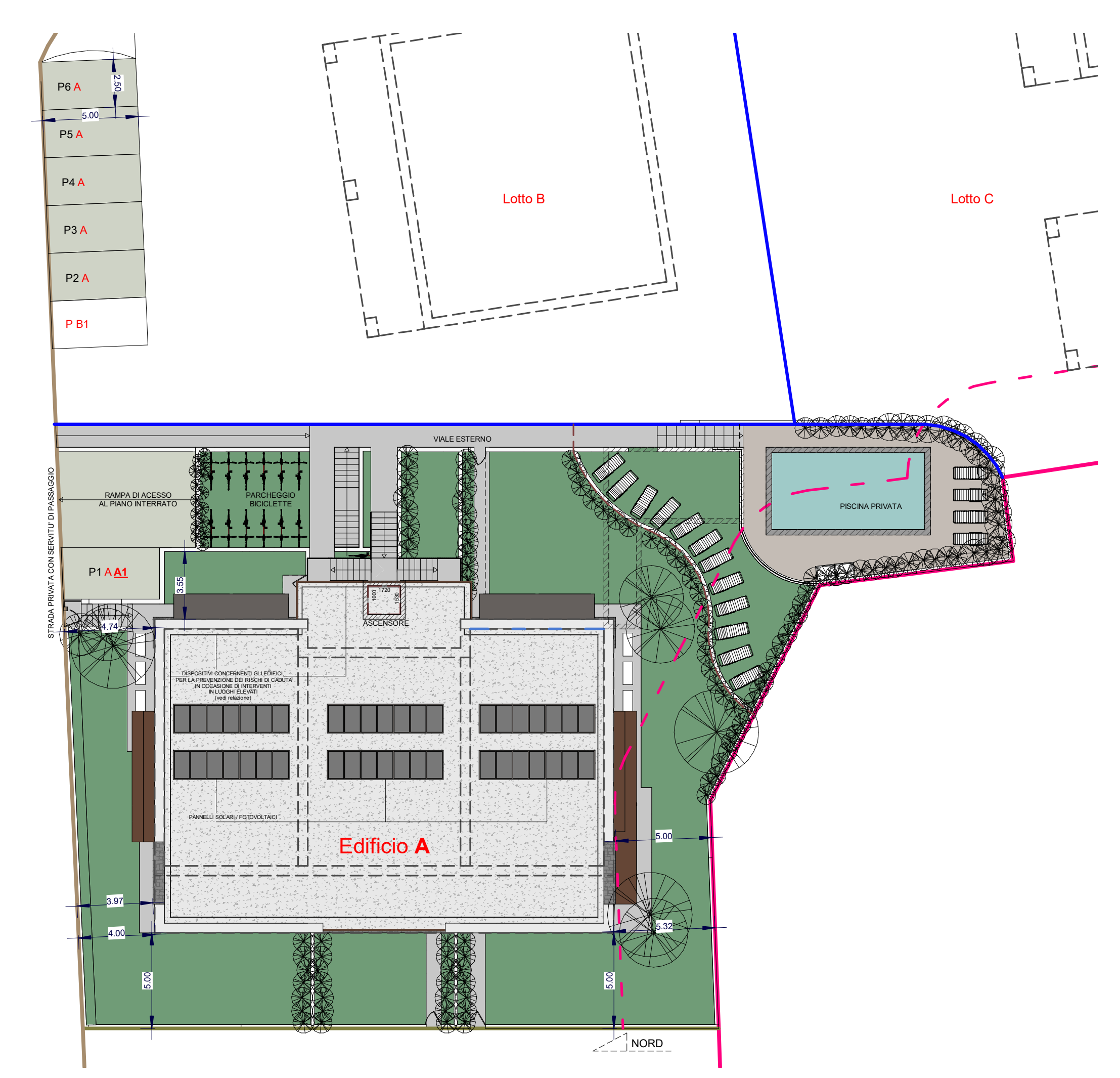
PLANIMETRIA GENERALE
